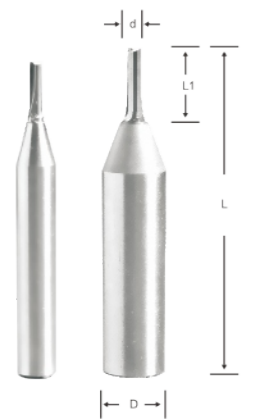
■ Carbide straight knife 合金直刀
