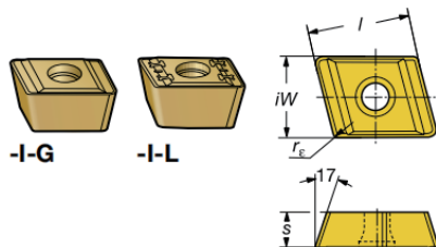
中间刀片
