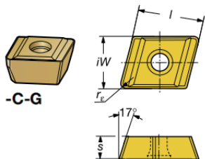
中心刀片
